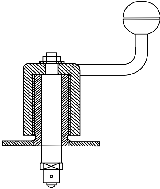
Manual Actuator
