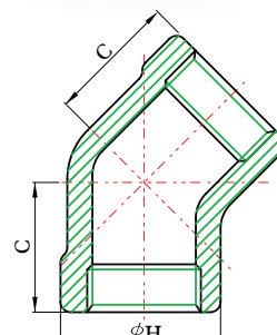
45° ELBOW
