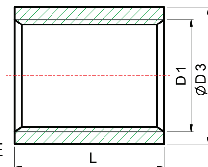
BSP, DIN 2999
